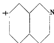
F oder \delta Säure.
